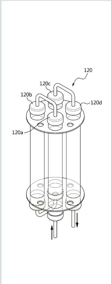
특허 10-1567699 회수헬륨 재사용 시스템에 사용되는 흡착탑 ▲
