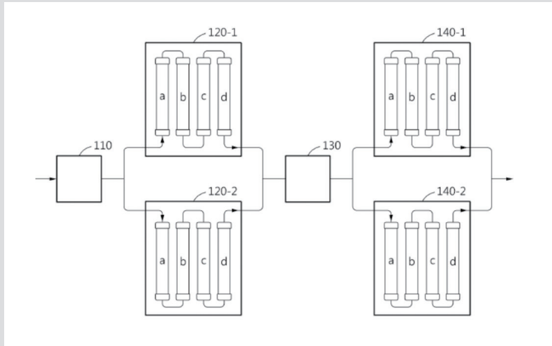
특허 10-1567699 회수헬륨 재사용 시스템의 블록도 ▲
